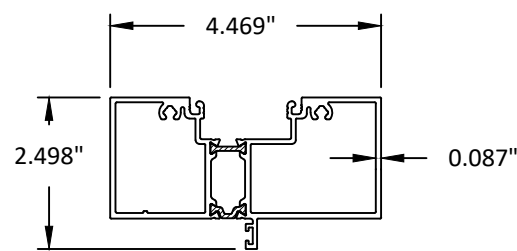
8 TRANSOM BAR
