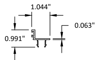
35 DOOR STOP
